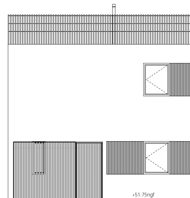
Façade Nord
