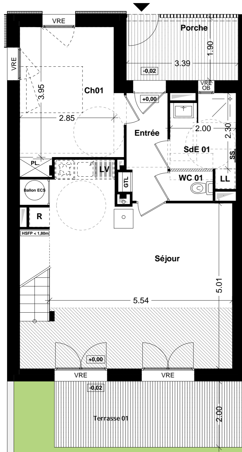
Rez-de-chaussée
