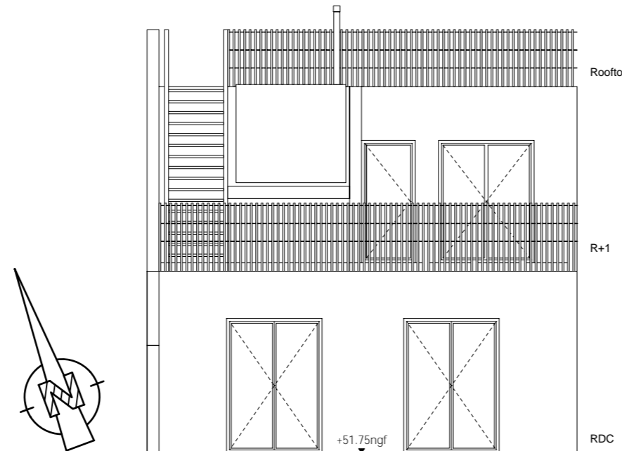
Façade Sud
