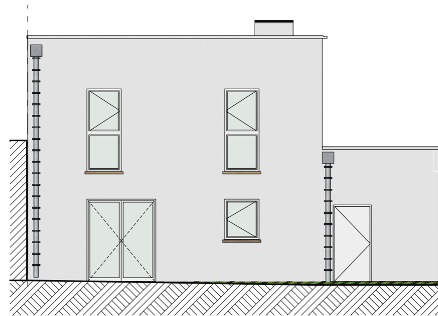
Façade Sud
