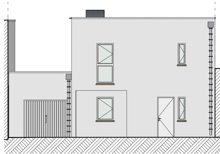
Façade Nord
